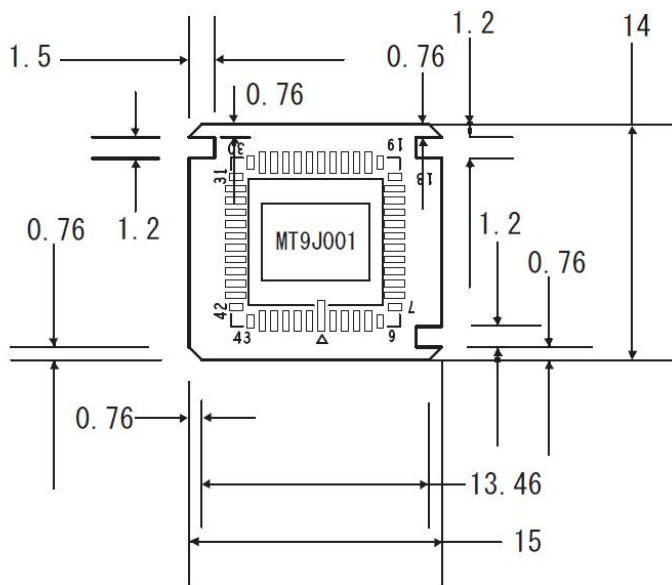
センサー基板：前面
