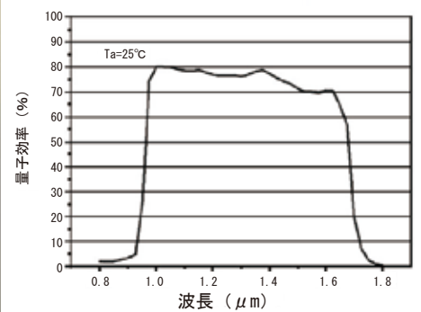
ARTCAM-008TNIR 代表的分光感度特性
